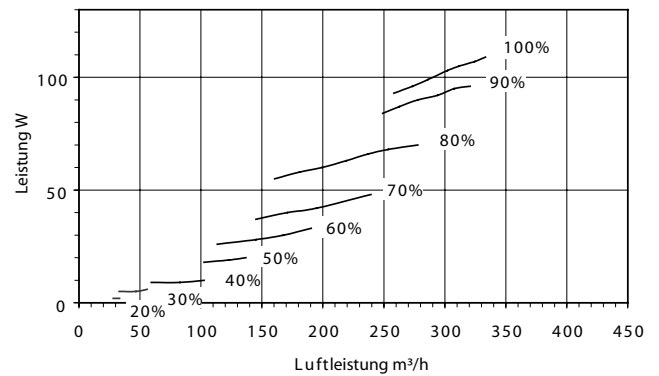
Pingvin eco ECE Gebläseleistung mit EU5 Vliesfilter
