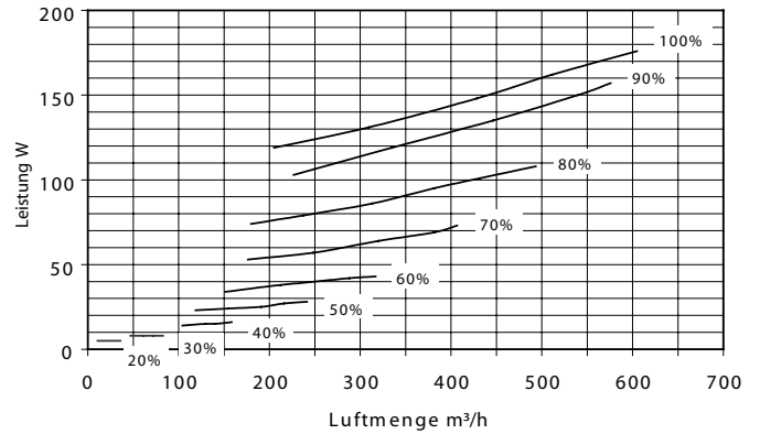
Pelican eco Gebläseleistung mit EU5 Taschenfilter
