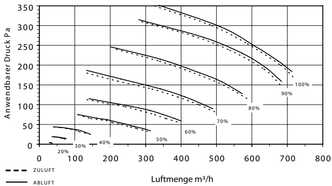
LTR-6-190 eco Zu- und Abluft Kennlinien mit F5 Filter
