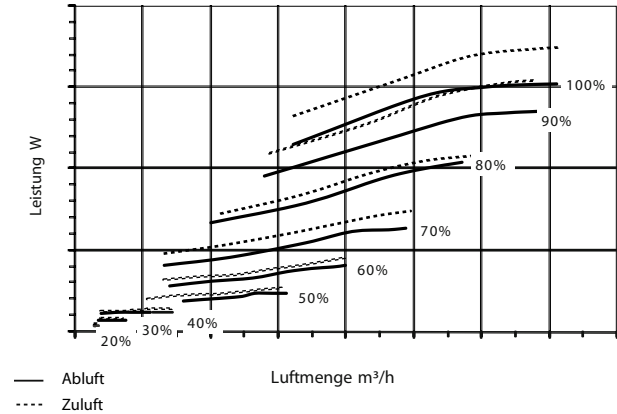
LTR-6 eco Gebläseleistung mit F5 Taschenfilter
