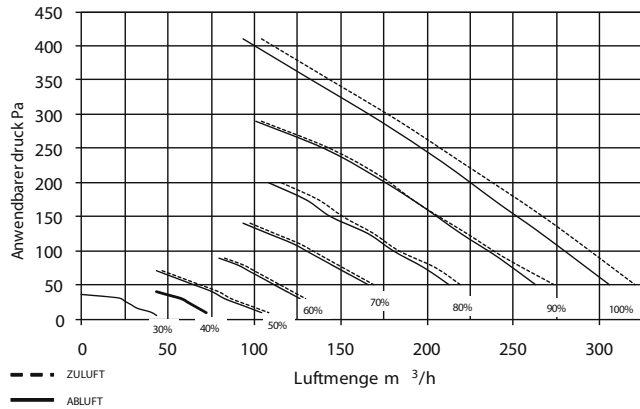
LTR-2 eco Zu- und Abluft Kennlinie mit F5 Filter
