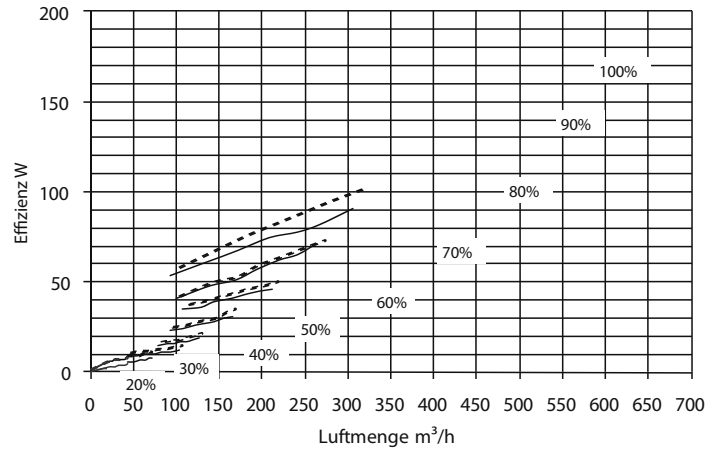
LTR-2 eco Gebläseleistung mit F5 Filter
